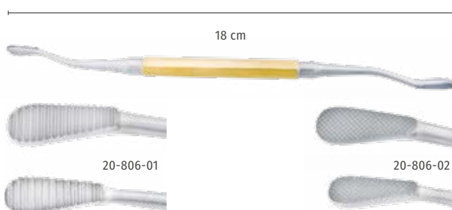
Miller Nasenraspel, Hartmetall, doppelseitig, 18 cm Miller nasal rasp, tungsten carbide, double ended, 18 cm
