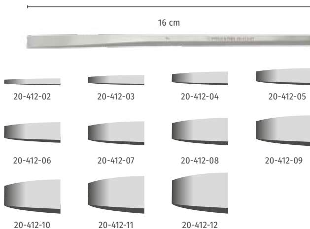
Rubin Osteotom, Sechskant-Griff, gerade, 16 cm
